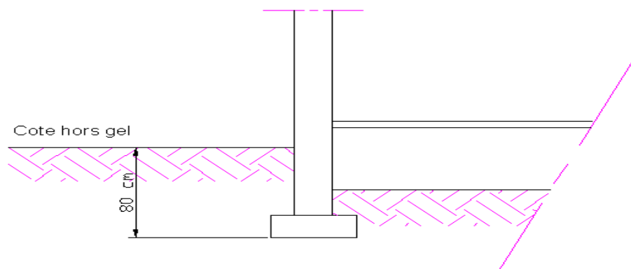
Profondeur d'ancrage des fondations
