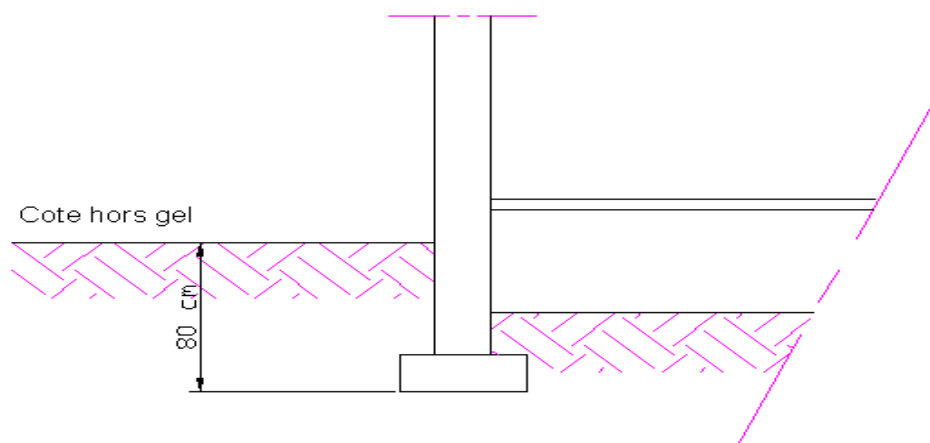
Profondeur d'ancrage des fondations
